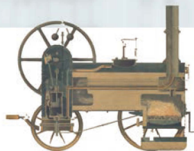
第四高等学校教育掛図 「モラン機械掛図 第28図 蒸気機関車」(附属図書館蔵)
